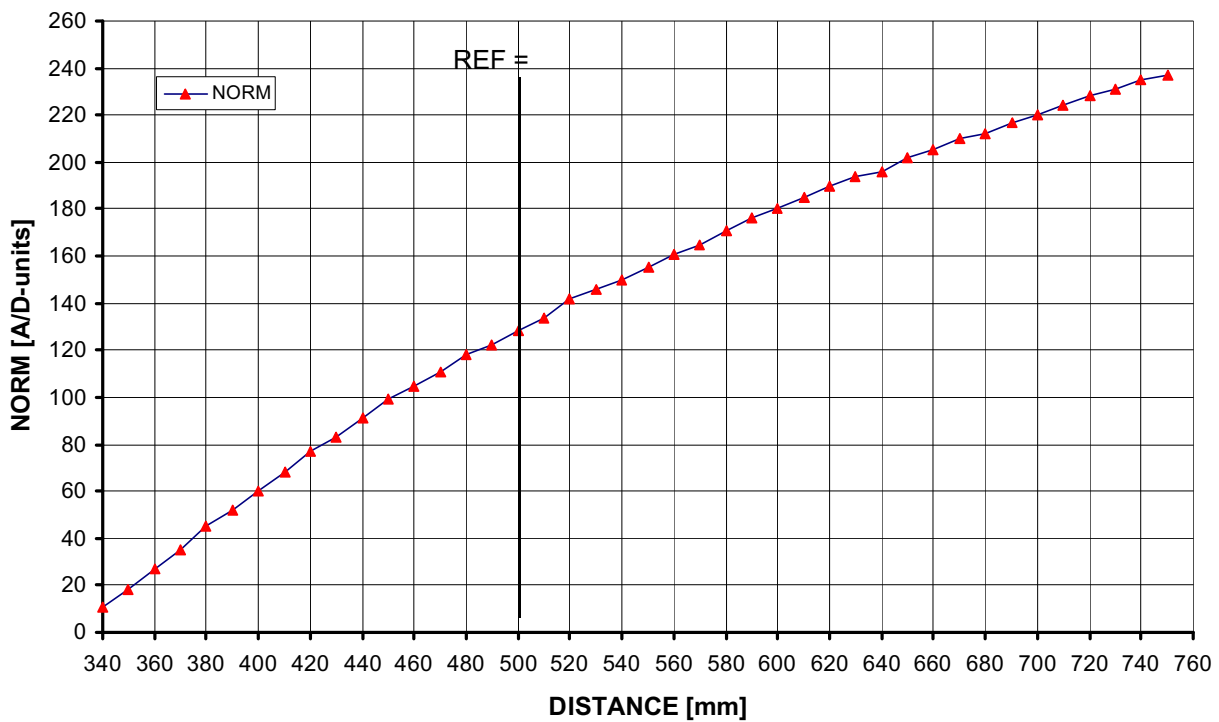
Characteristic Curve: R-LAS-LT-500-XL-ANA (Ser.No. 00878)
