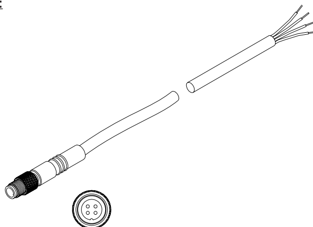
Anschlusskabel zur SPS: cab-M5/4-g-2
