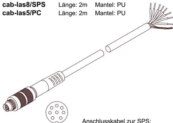
Anschlusskabel zur SPS: cab-las8/SPS
