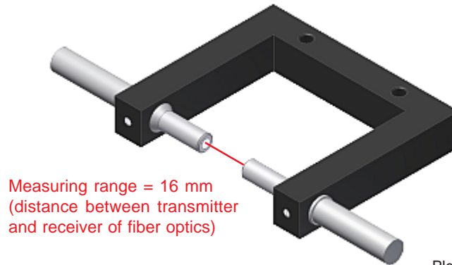
C-MOUNT-A3.0-180°-16/50
